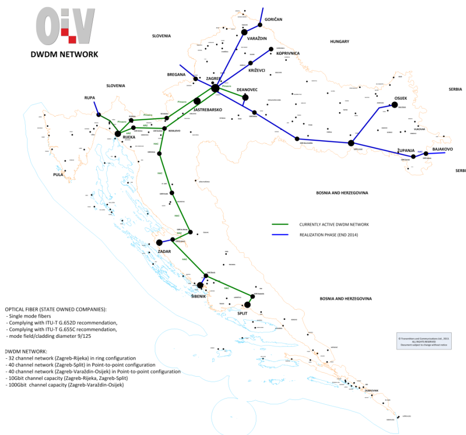
Slika 5-3 DWDM mreža – postojeće stanje i plan proširenja
