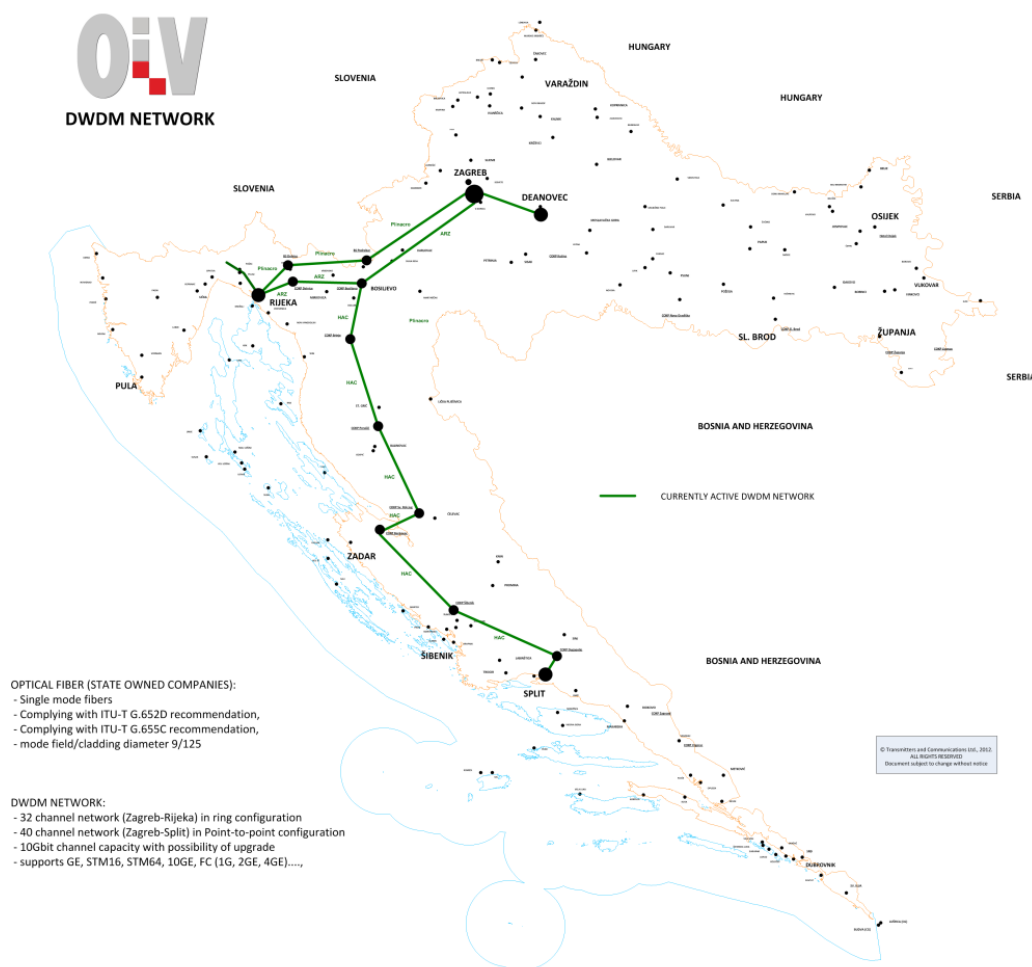
Slika 5-2 DWDM mreža – postojeće stanje
