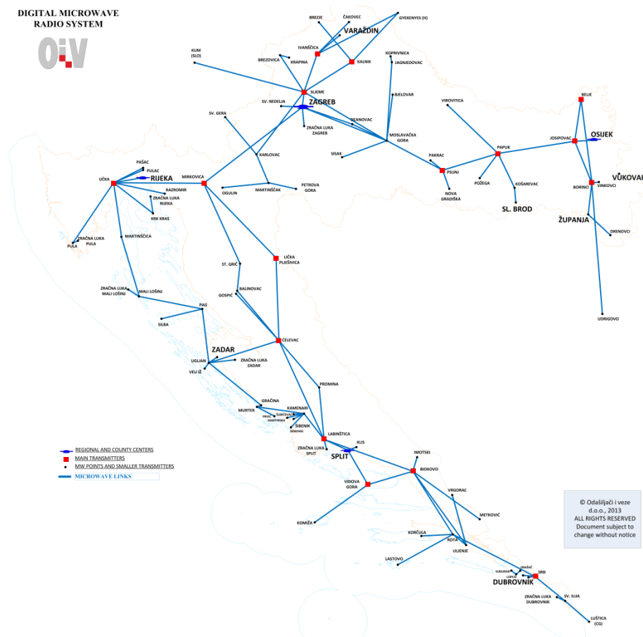
Slika 5-4 Mikrovalna OiV mreža
