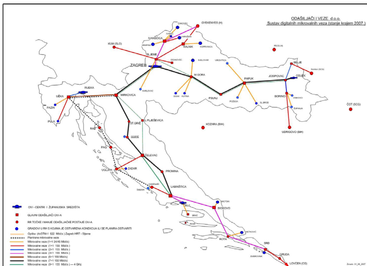
Grafički prikaz 15. Karta veza s 4 GHz kao stanje 31.12.2007.
