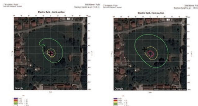
Fotografija: Spectrum lab, EM proračun DAB Autor: Jasminka Cigrovski
